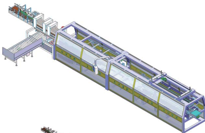
LP-ZX-60TB Encajonadora wrap-around
