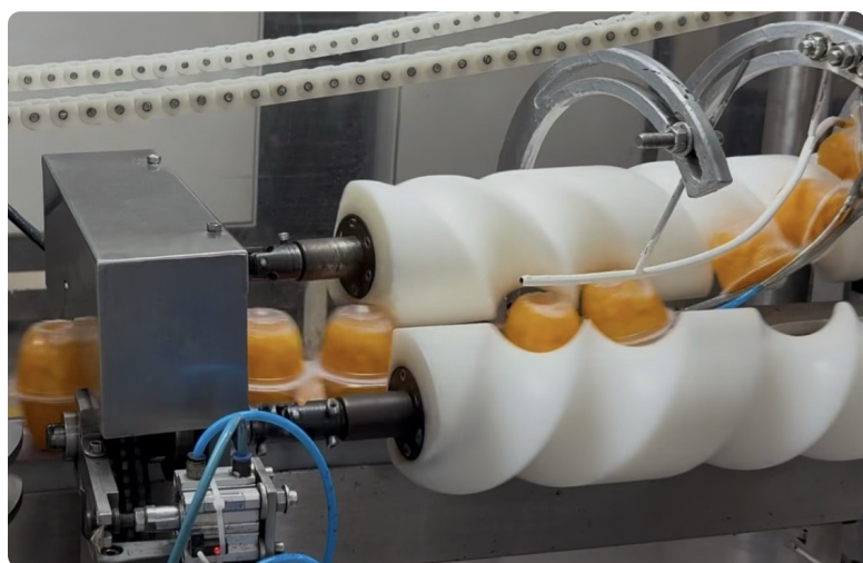
Dos tornillos sinfín apilan los vasos boca a boca antes del enfajado
